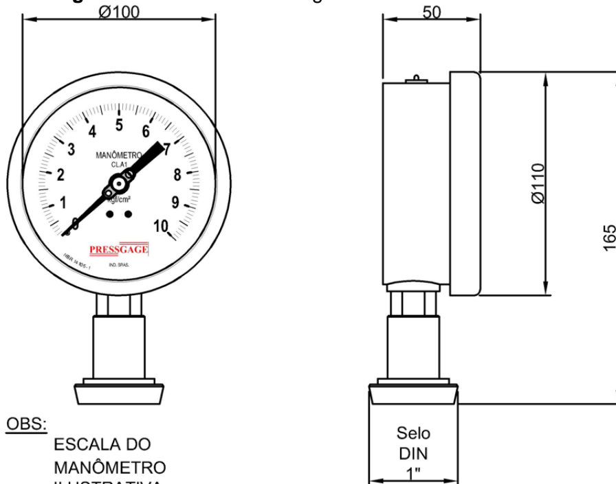
Figura 3 – Manômetro analógico Ø100mm com selo DIN
