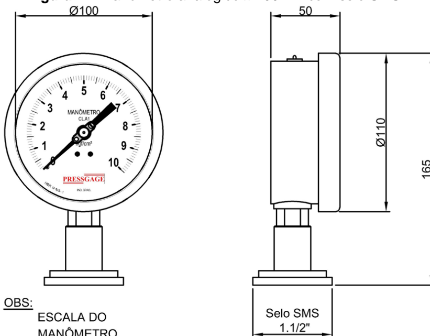
Figura 4 – Manômetro analógico Ø100mm com selo SMS
