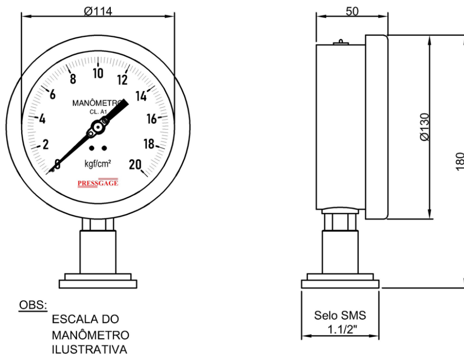
Figura 6 – Manômetro analógico Ø114mm com selo SMS
