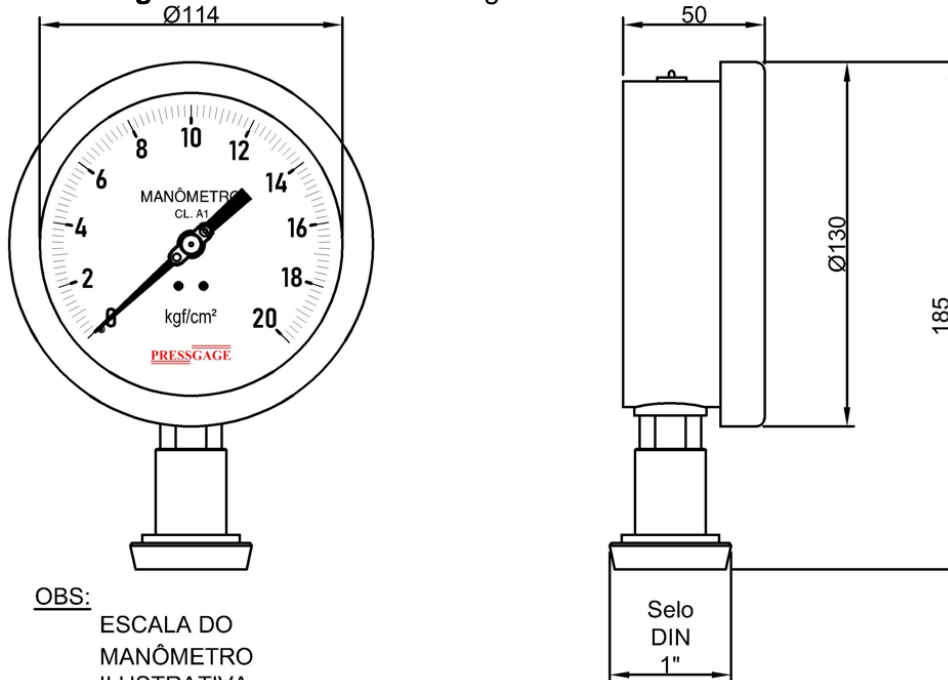
Figura 5 – Manômetro analógico Ø114mm com selo DIN
