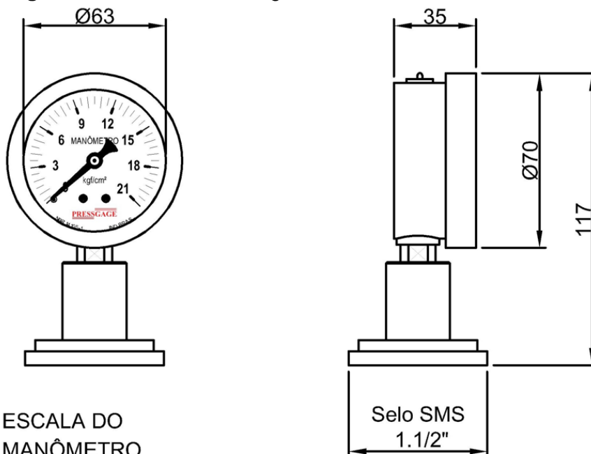
Figura 2 – Manômetro analógico Ø63mm com selo SMS
