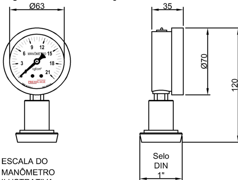
Figura 1 – Manômetro analógico Ø63mm com selo DIN
