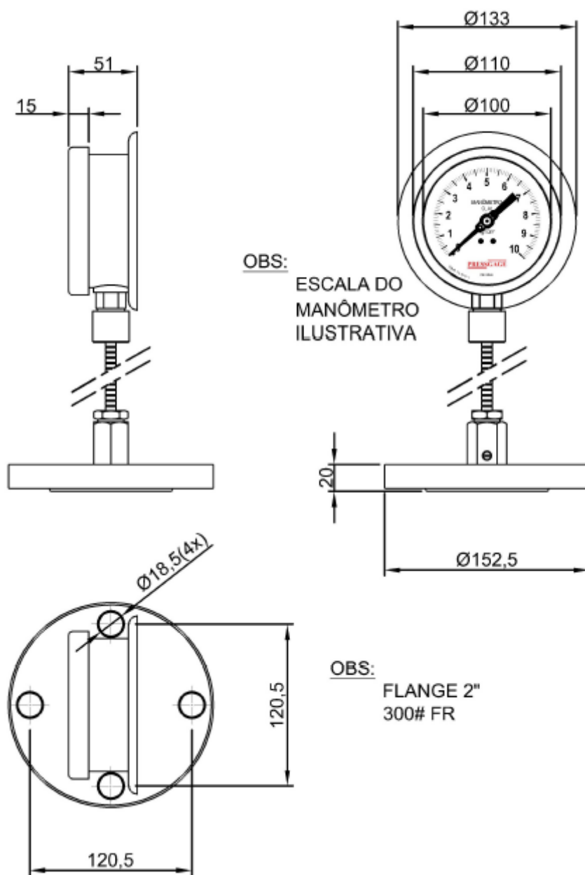
Figura 1: Manômetro analógico Ø100mm com selo flangeado e capilar
