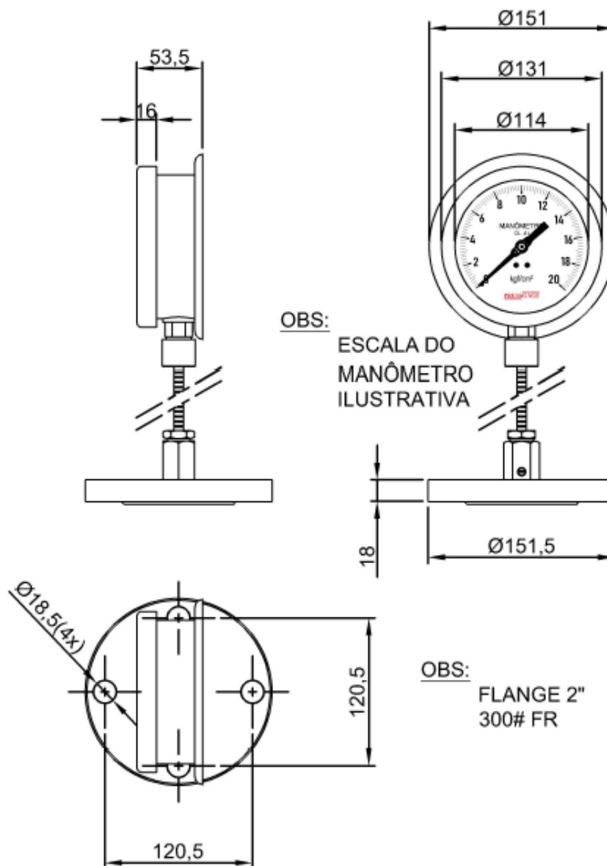
Figura 2: Manômetro analógico Ø114mm com selo flangeado e capilar
