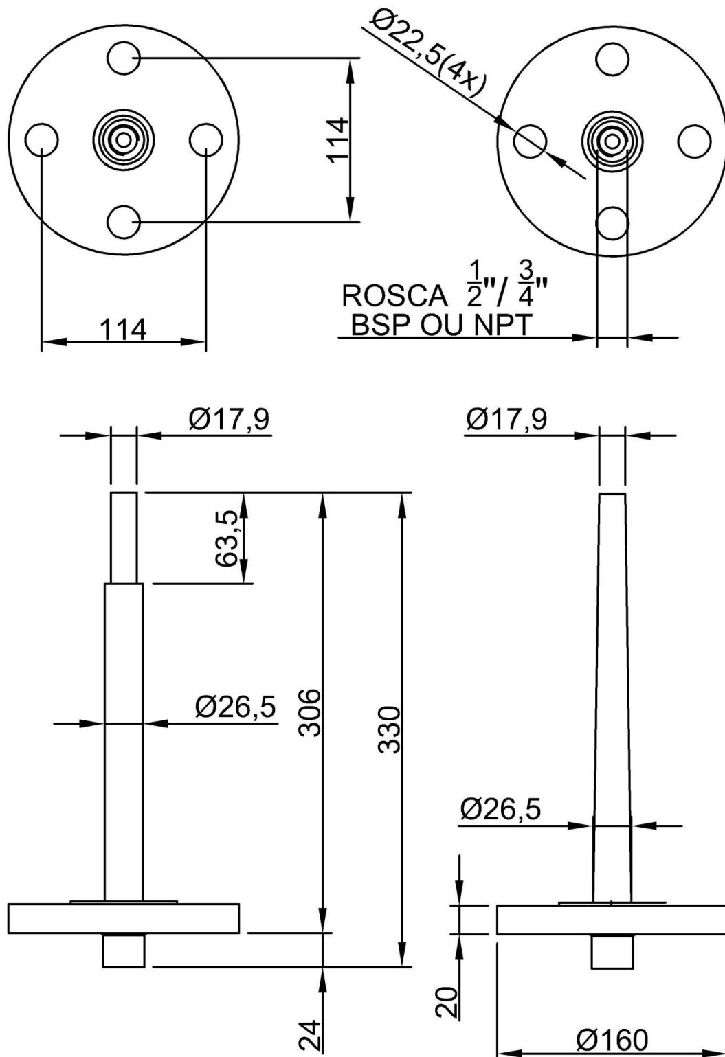
Figura 1: Poço flangeado
