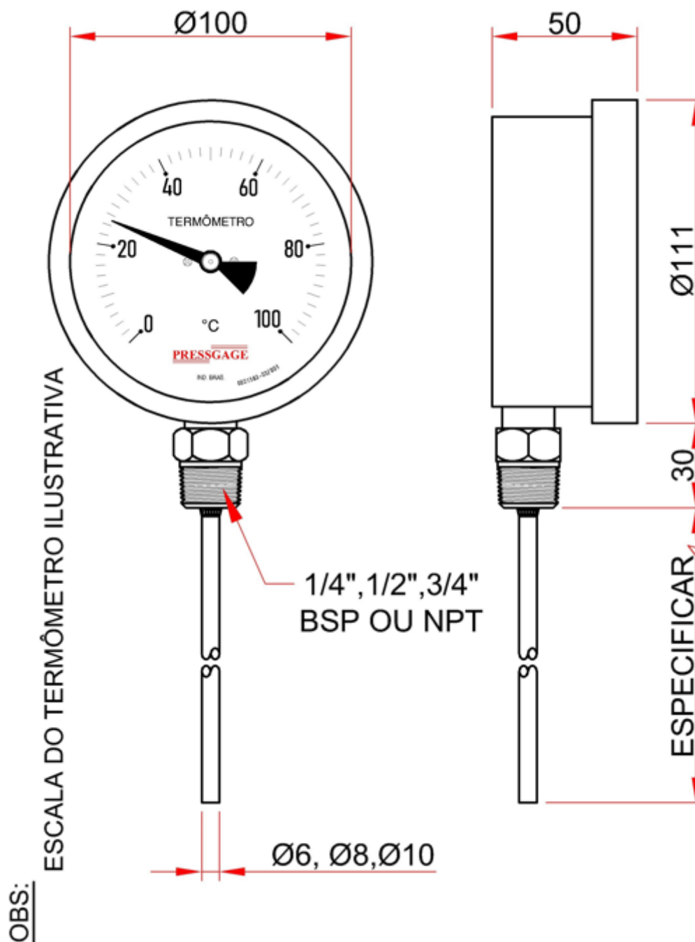
Figura 2 – Termômetro analógico vertical Ø100mm
