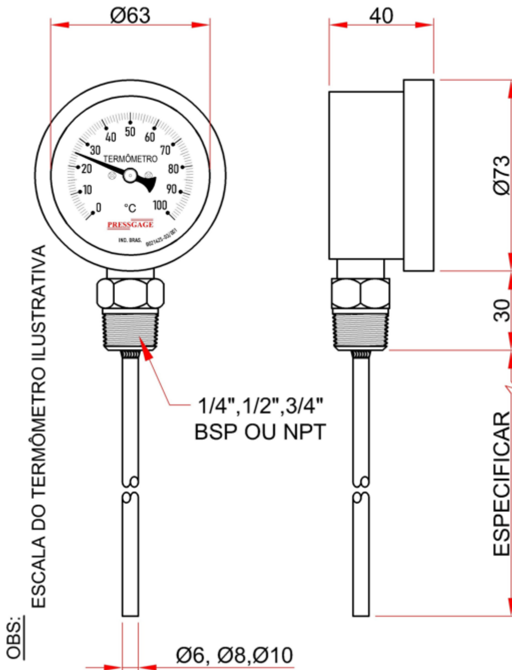
Figura 1 – Termômetro analógico vertical Ø63mm
