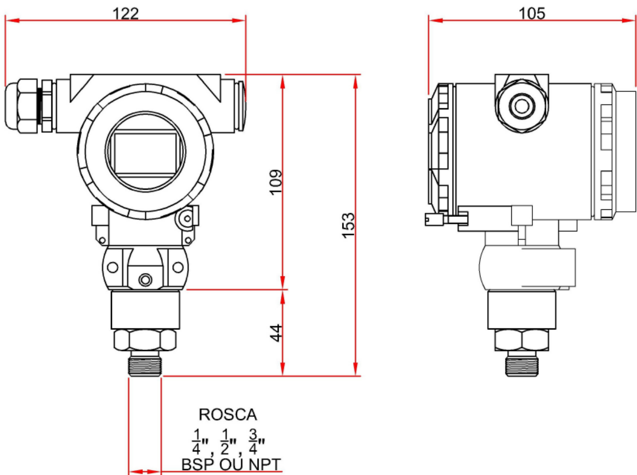
Figura 1: Transmissor de pressão com protocolo HART
