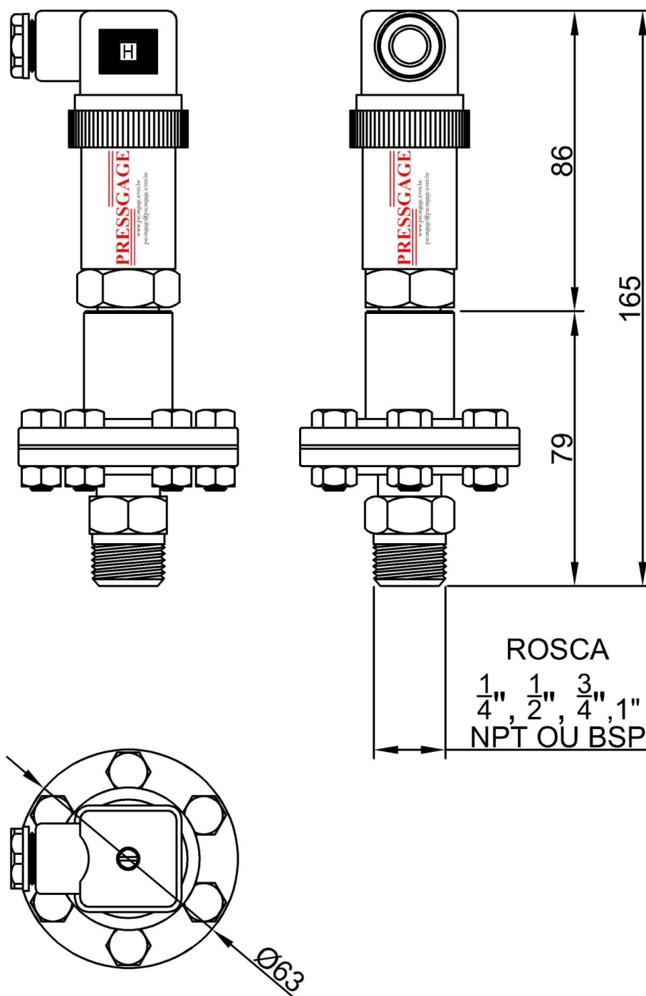
Figura 1: Transmissor de pressão com selo diafragma
