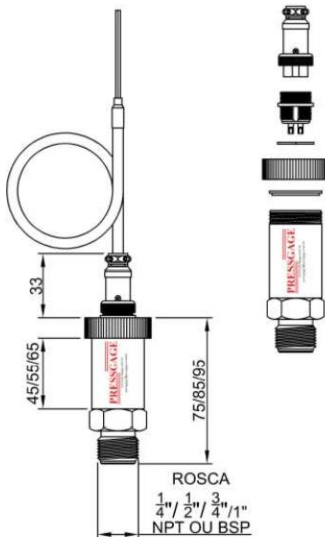
Figura 1: Transmissor de pressão com conector M12
