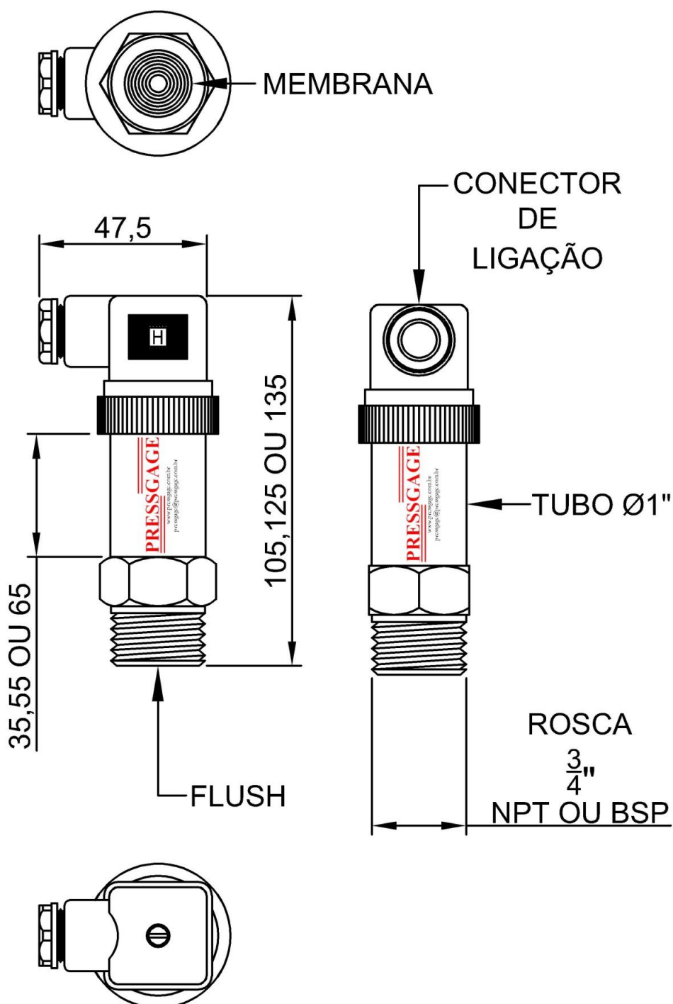
Figura 1: Transmissor de pressão com conexão flush
